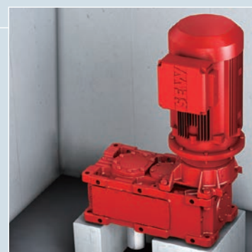
モータアダプター付
