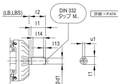
C：反負荷側延長軸寸法
