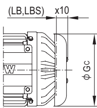
B：防滴キャノピ追加寸法
