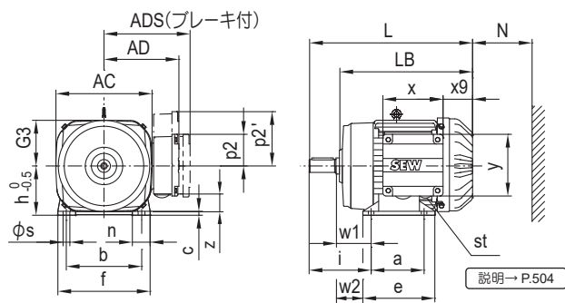
DRN71 - 132S
