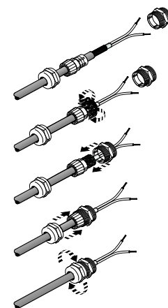
ケーブルグランドとシールドケーブル
