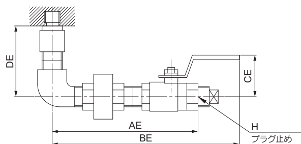
エルボ型ドレンバルブ
