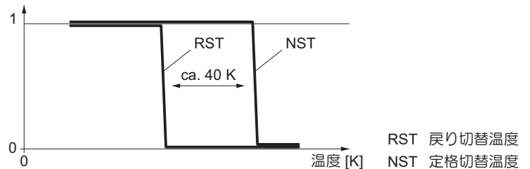
サーモスタット「ブレーク接点」の切替状態：
