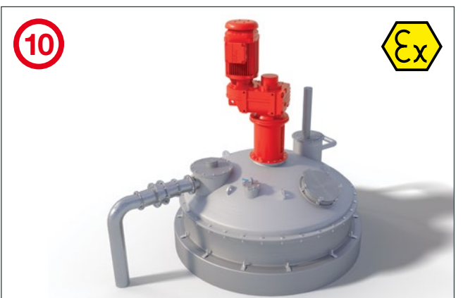
Faulturm Unser Lösungsbeispiel: Flachgetriebemotor F..DR.. als Rührwerksausführung mit verlängertem Lagerabstand.
